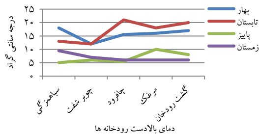
شکل ۳: تغییرات درجه حرارت آب در بالا دست رودخانه‌های حوزه تالاب انزلی در فصول مختلف
