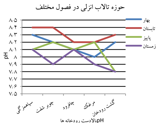
شکل ۶: تغییرات pH آب بالادست رودخانه‌های حوزه تالاب انزلی در فصول مختلف
