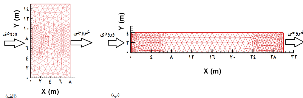
شکل ۴: محیط فیزیکی گسسته‌سازی شده مربوط به دو حوضچه مستطیلی؛ الف) B با ضریب هندسی ۰/۵۳ و ب) G با ضریب هندسی ۷/۵
