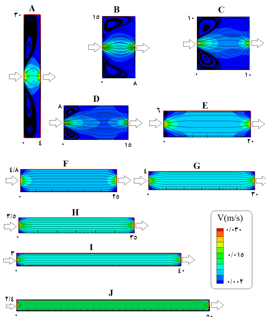
شکل ۶: نتایج شبیه‌سازی شده در قالب خطوط جریان و مناطق هم‌سرعت جریان در حوضچه‌های فرضی ده‌گانه
