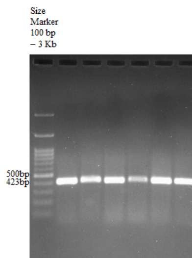
شکل ۲: نتیجه واکنش PCR بر روی ژن تیروزیناز ماهی قزل آلائی رنگین کمان (پرایمرهای اختصاصی این ژن توانسته اند قطعات ۴۲۳ جفت باز را تکثیر دهند)
