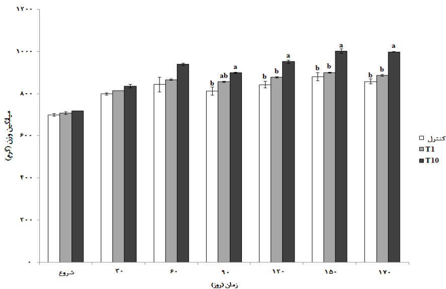
شکل ۲: روند تغییرات وزن بدن مولدین استرلیاد تحت تزریق غلظت مختلف هورمون تیروکسین طی آزمایش ۱۷۰ روزه (میانگین \pm خطای استاندارد). حروف متفاوت بیانگر اختلاف معنادار در بین تیمارهای مختلف در زمان‌های مختلف است ( p < 0.05 ).
