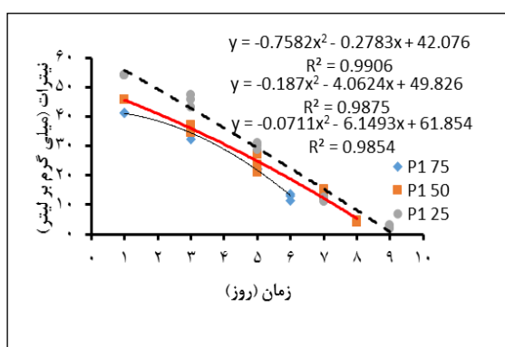
شکل ۱: میزان نیترات اندازه‌گیری شده در طول آزمایش در غلظت‌های مختلف p_1 و p_2
