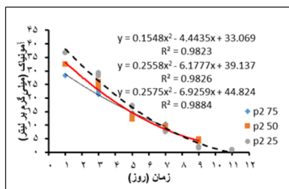
شکل ۳: میزان آمونیاک اندازه‌گیری شده در طول آزمایش در غلظت‌های مختلف P ۱ و P ۲
