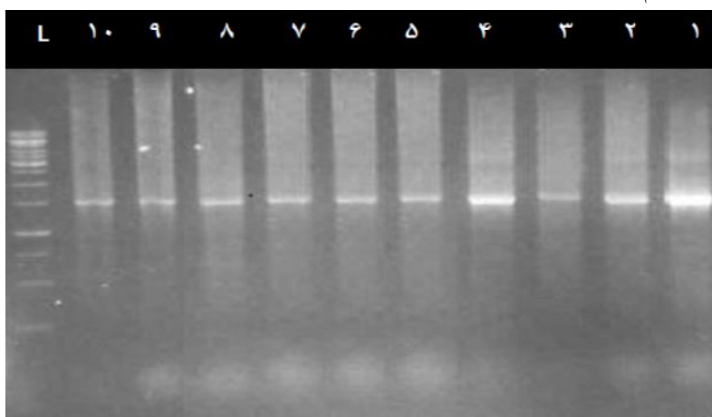
شکل ۱: قطعات تکثیری توالی های 16s rDNA ایزوله ها با استفاده از جفت آغاز گرهای اختصاصی
