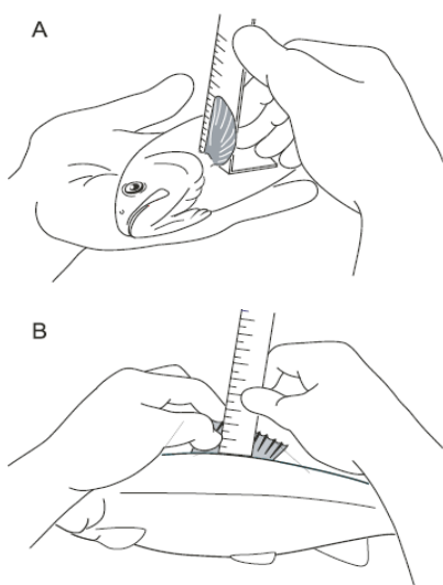
شکل ۱: نحوه اندازه‌گیری حداکثر ارتفاع باله‌ها. A: باله سینه‌ای چپ، B: باله پشته (Person-Le Ruyet et al., 2007)
