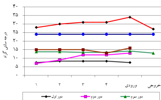
شکل ۲: تغییرات دمای هوا در دریاچه سد گلابر زنجان
