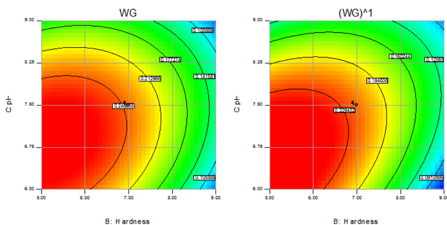
شکل ۶: نمودار دو بعدی متغیر سختی و pH برای تعیین نقطه بهینه دما در افزایش وزن ماهی آنجل در بازه زمانی دوم
