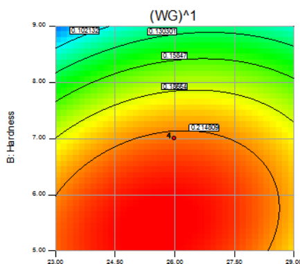
شکل ۱: نمودار دو بعدی متغیر دما و سختی برای تعیین نقطه بهینه pH در افزایش وزن ماهی آنجل در بازه زمانی اول
