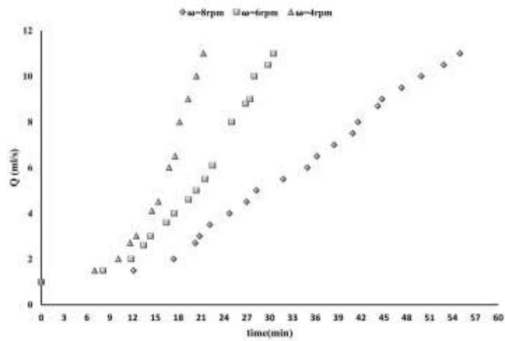
شکل ۳ الف: نمودار افت-زمان برای دبی ورودی ۵۵۰ میلی‌لیتر بر ثانیه (سطح غرقابی ۱۵ درصد و غلظت ۳۰ میلی‌گرم بر لیتر) در سرعت‌های چرخشی ۸ دوربر دقیقه ( SEM^4=0.051 )، ۶ دوربر دقیقه ( SEM=0.06 ) و ۴ دوربر دقیقه ( SEM=0.058 ).
